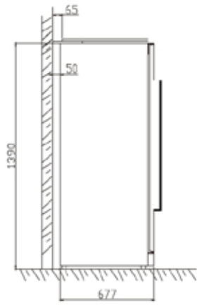
安裝側視圖
