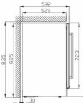
安裝側視圖
